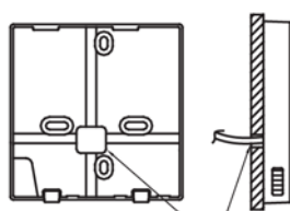
Foro nel muro e per i fili Diametro foro: \varnothing 20\text{mm}
