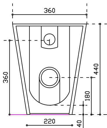
Vista posteriore
