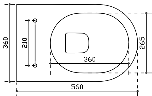
Vista dall'alto
