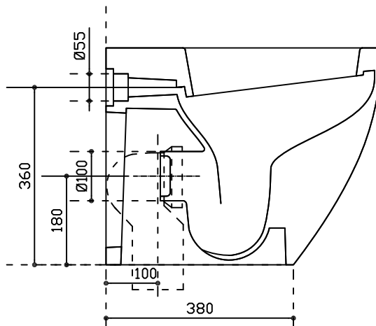
Sezione
