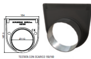
TESTATA CON SCARICO 150/160
