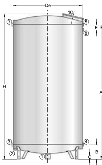
PASSO D'UOMO DECENTRATO PER CAPACITÀ DA 3000 A 15000 LITRI
