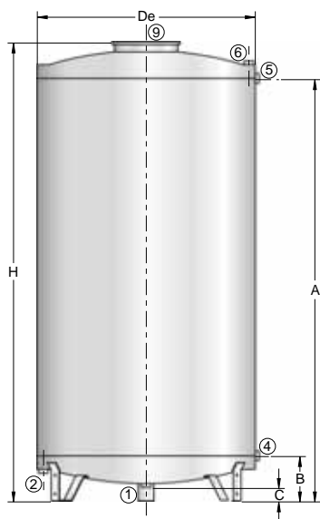
PASSO D'UOMO CENTRATO SULL'ASSE PER CAPACITÀ DA 125 A 2000 LITRI
